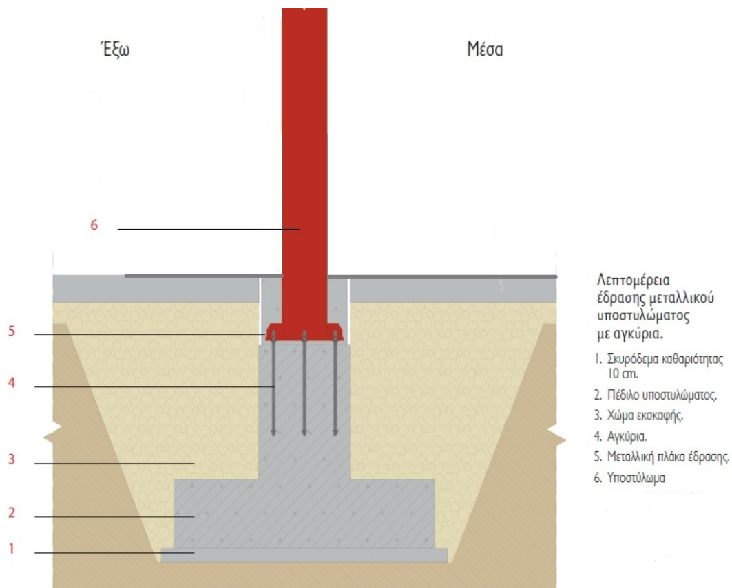
Σκίτσο Τοποθέτησης Υποστυλώματος
